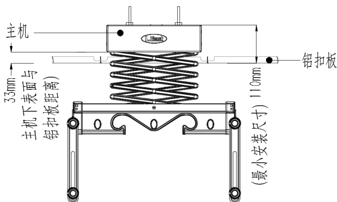
安装总图
